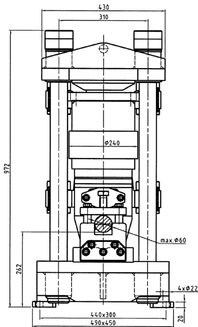
Fig.1 Dimensiunile de gabarit ale preseii hidraulice de debitat HPHD-200.060
